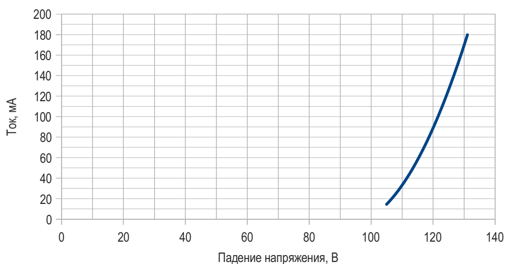
Вольт-амперная характеристика
