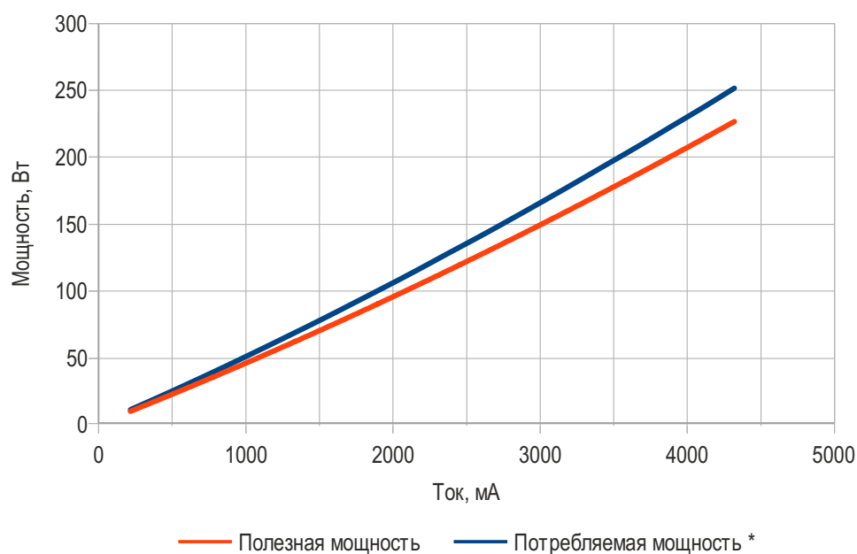
График зависимости полезной и потребляемой* мощностей от поданного тока
